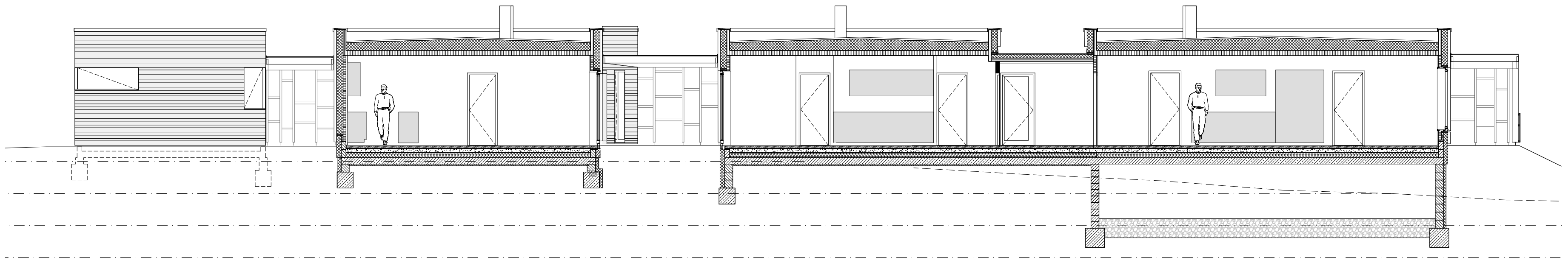
LÄNGSSCHNITT
