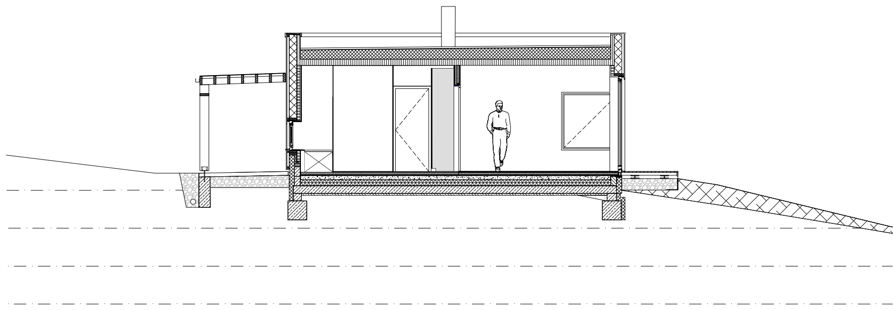
QUERSCHNITT HAUS MEDIUM
