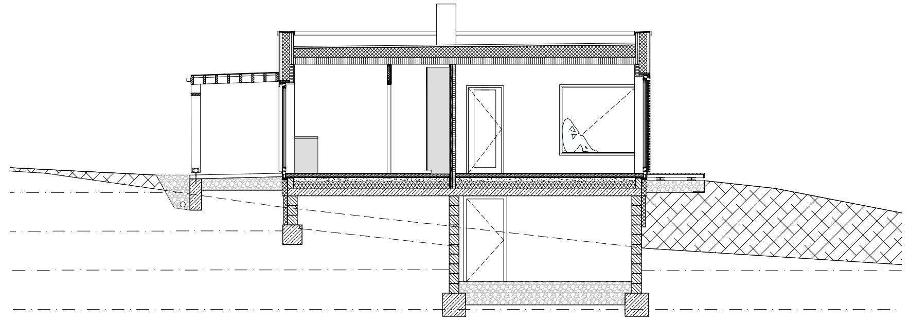
QUERSCHNITT HAUS LARGE MIT ERDKELLER
